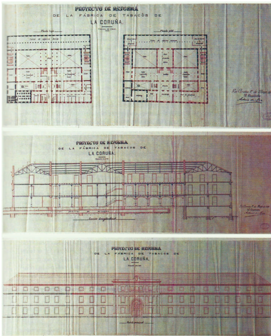
Planta, alzado e fachada da reforma da Fábrica de Tabacos. 1908. AMC.
